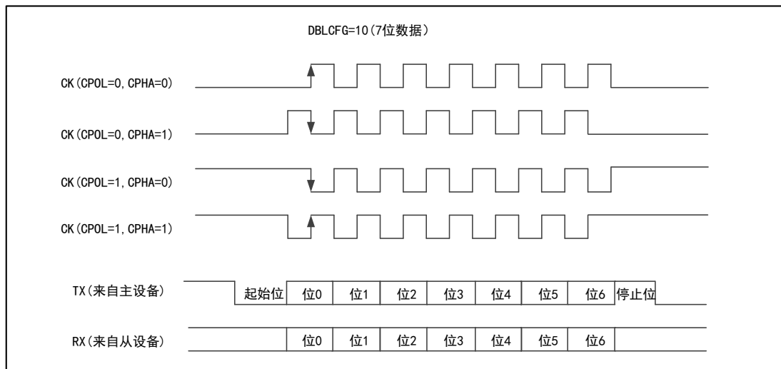
图 88 USART 同步传输时序图 (DBLCFG=10)
