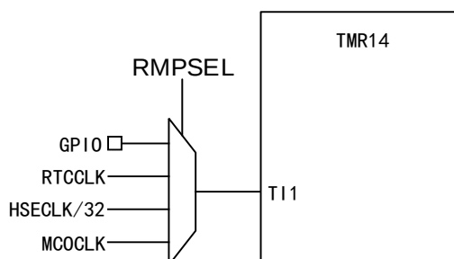
图 6 TMR14 间接测量时钟频率电路图
