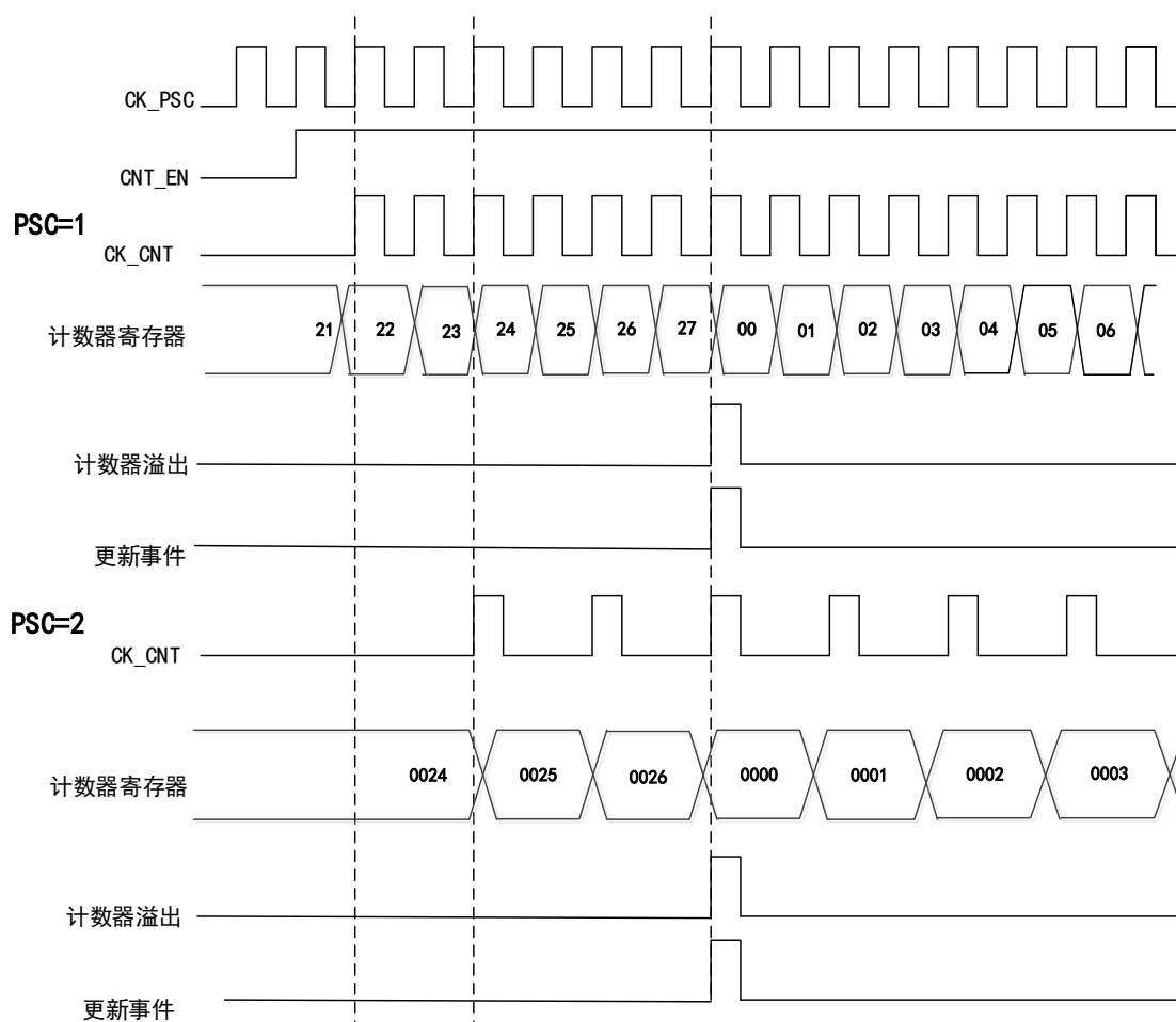
图 67 向上计数模式下，分频因子为 1 或 2 的时序图
