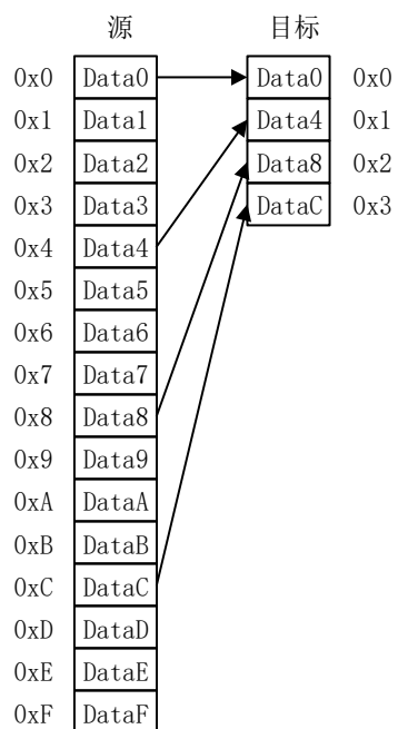
图 12 源为 32bits 目标为 8bits 的传输宽度
