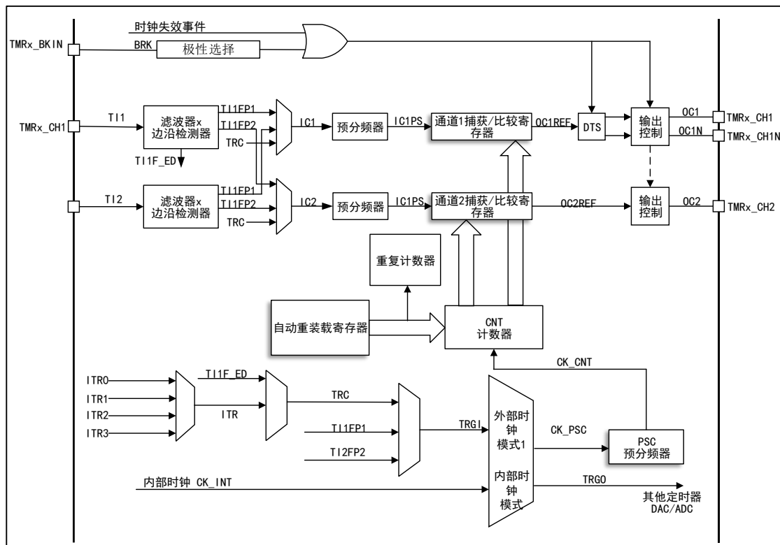
图 65 通用定时器 TMR15 结构框图
