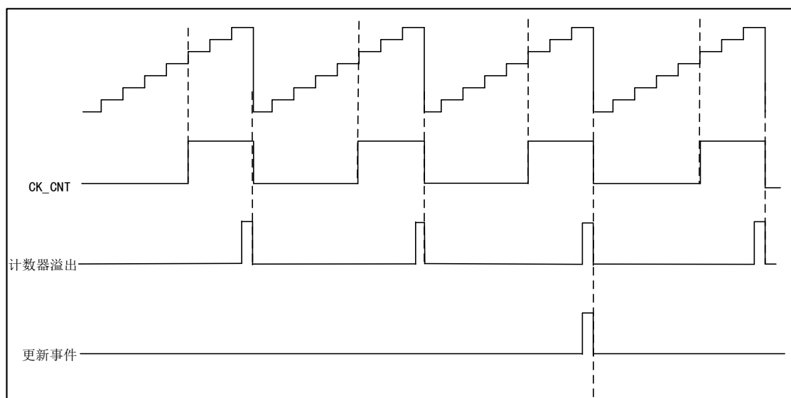
图 68 向上计数模式下，设置 REPCNT=2 的时序图
