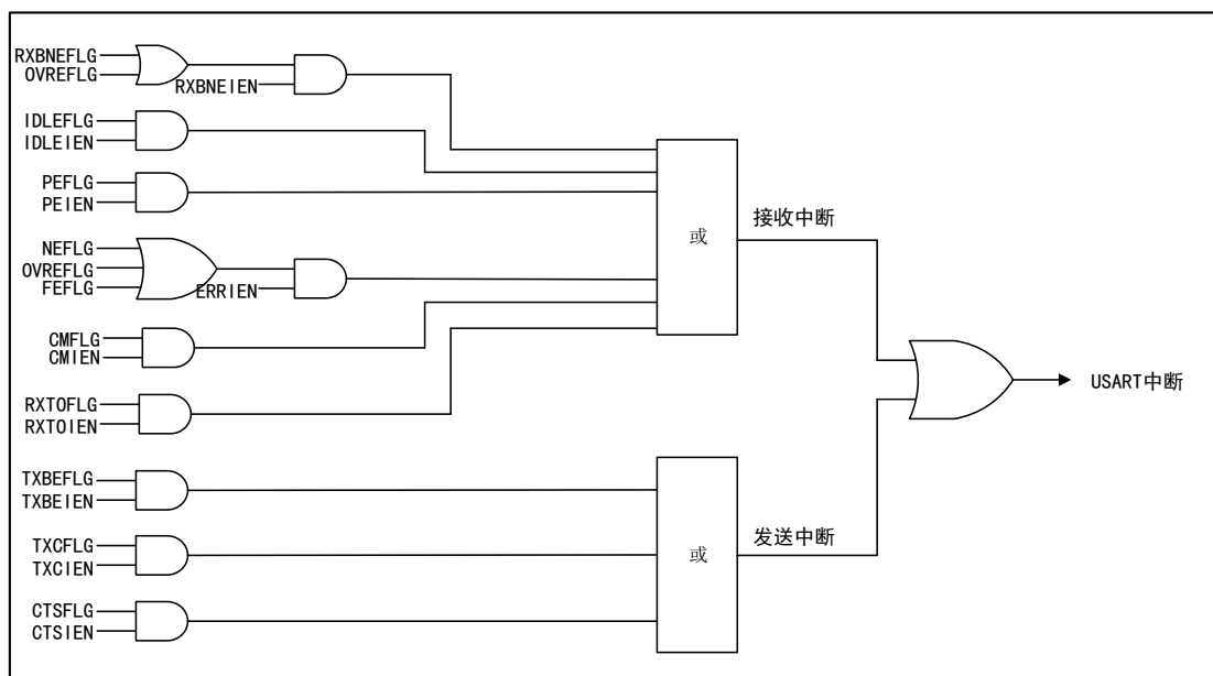
图 92 USART 中断映射
