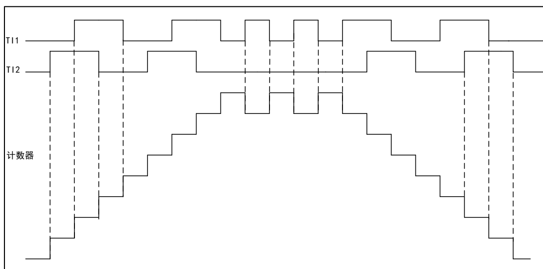
图 56 编码器模式下的计数器操作实例
