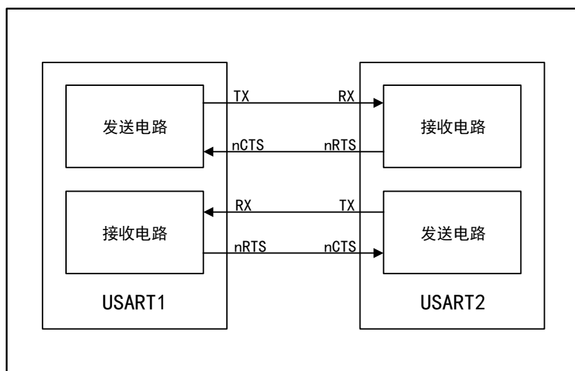
图 91 两个 USART 之间的硬件流控制
