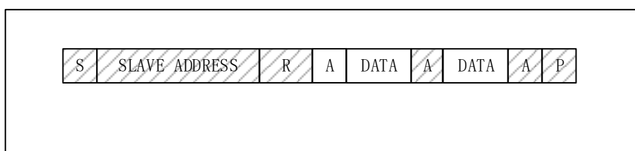
图 97 主机由从机读取数据
