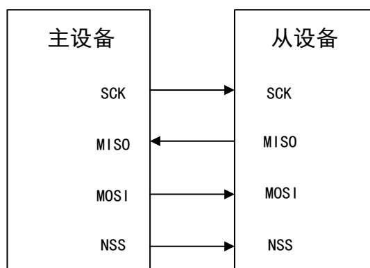
图 100 半双工模式连接
