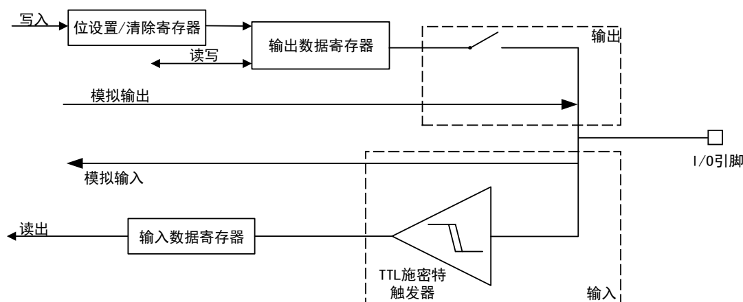
图 21 模拟功能 I/O 结构
