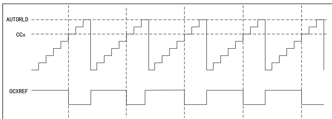
图 69 PWM1 向上计数模式的时序图
