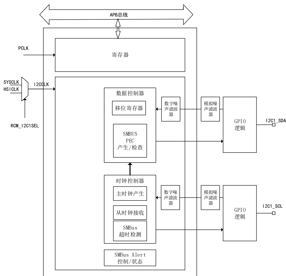
图 93 I2C1 功能结构图
