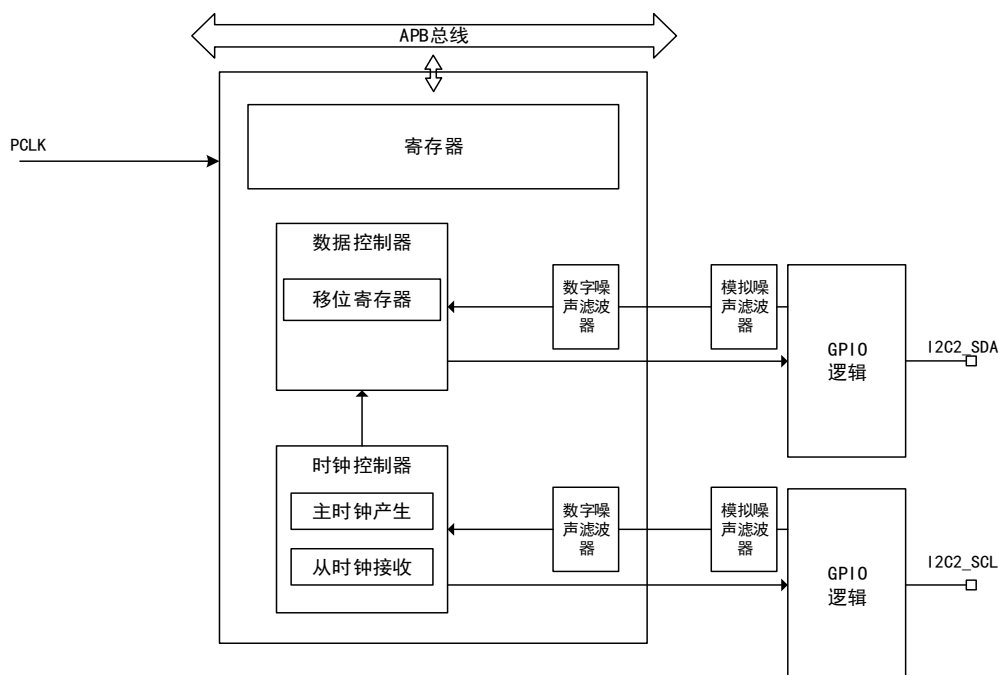
图 94 I2C2 功能结构图
