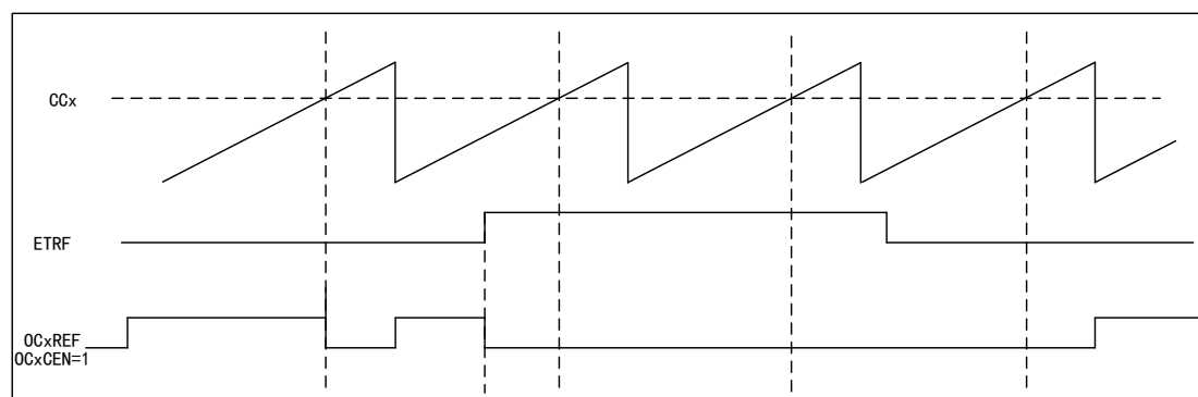
图 43 OCxREF 时序图
