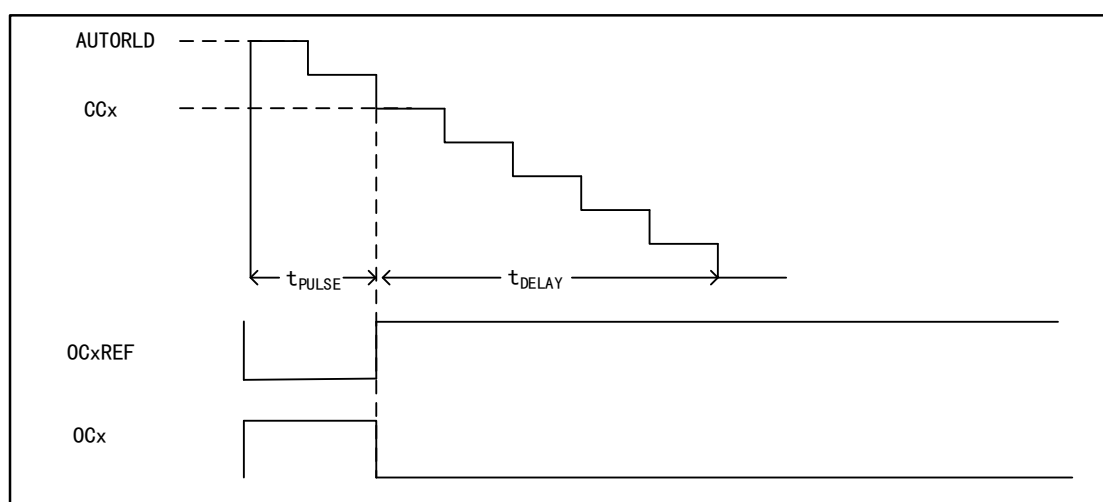
图 72 单脉冲模式下的时序图
