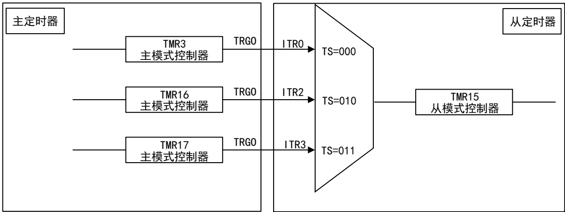
图 76 TMR15 与其它定时器互连
