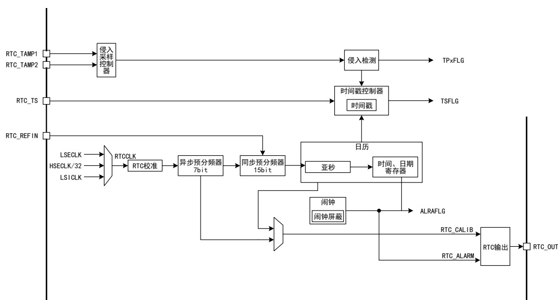
图 83 APM32F030x6x8 RTC 结构框图
