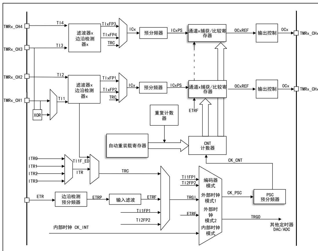
图 44 通用定时器 TMR3 结构框图
