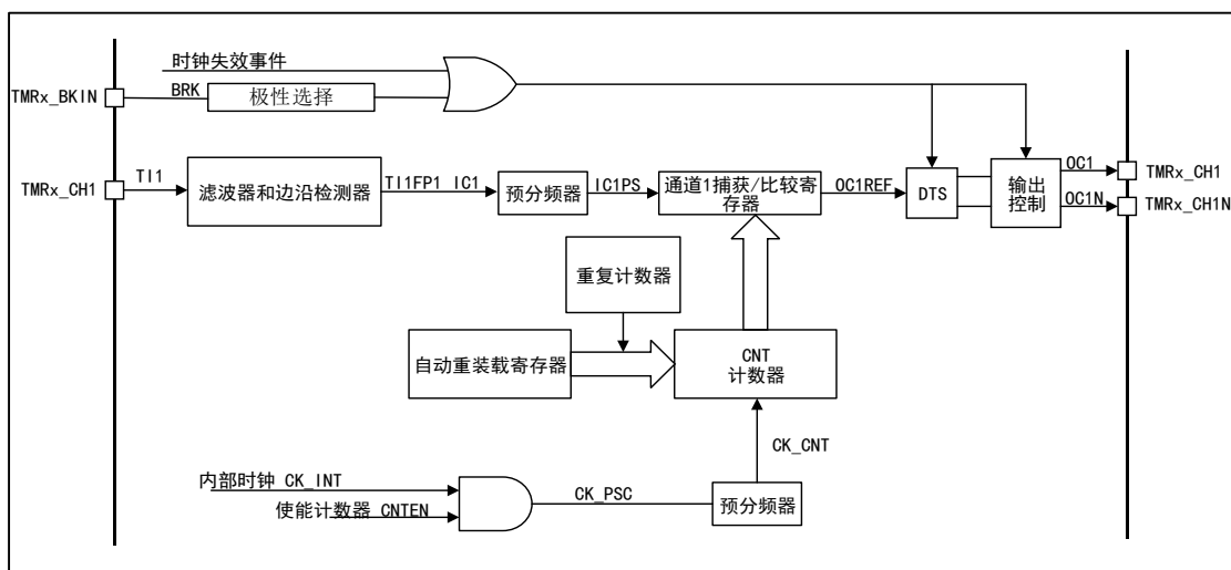
图 66 通用定时器 TMR16/17 结构框图
