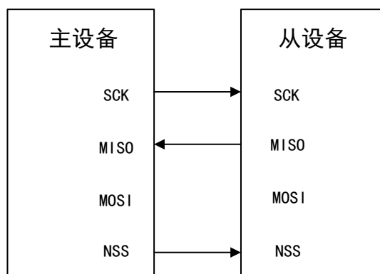
图 101 单工模式连接（主机用来接收，从机用来发送）
