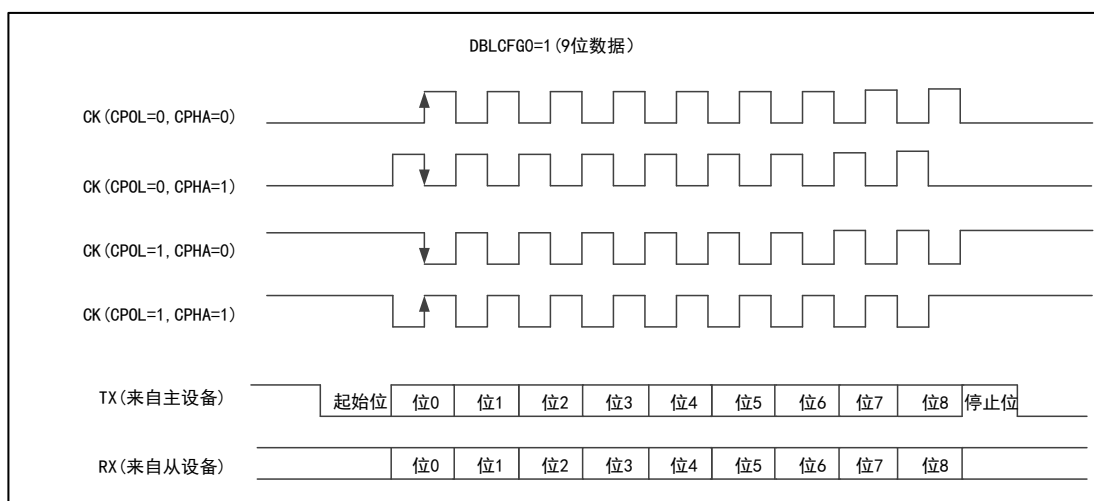
图 90 USART 同步传输时序图 (DBLCFG0=1)
