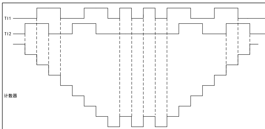
图 57 TI1FP1 反相的编码器接口模式实例
