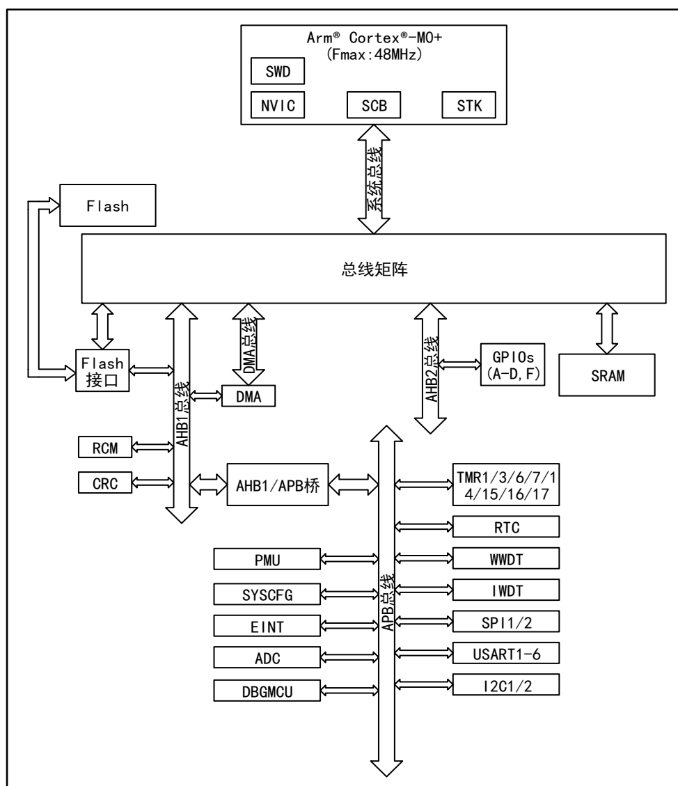
图 1 APM32F030x6x8xC 系统架构框图
