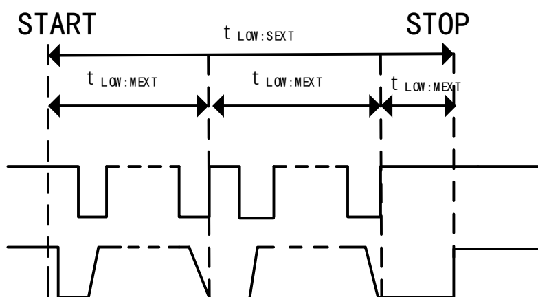
图 98 t_{\text{LOW:SEXT}} 与 t_{\text{LOW:MEXT}} 时间
