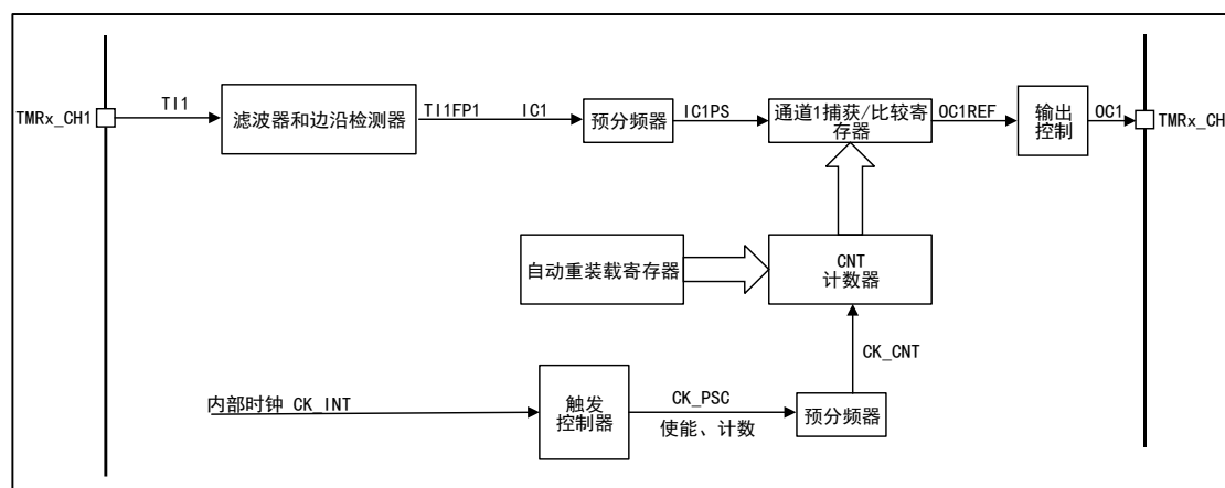
图 61 通用定时器 TMR14 结构框图
