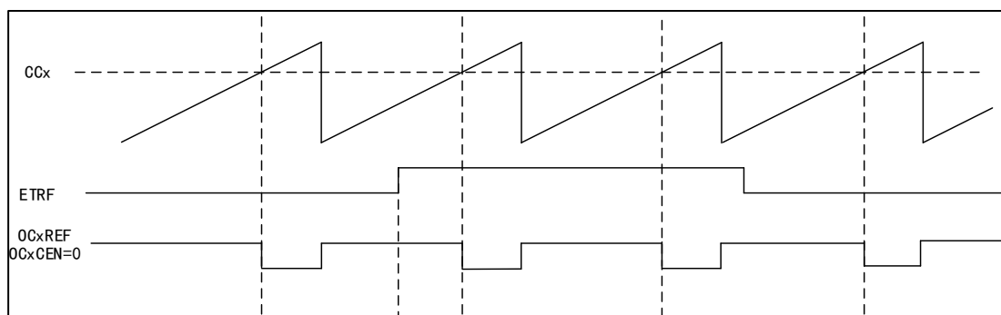
图 59 OCxREF 时序图
