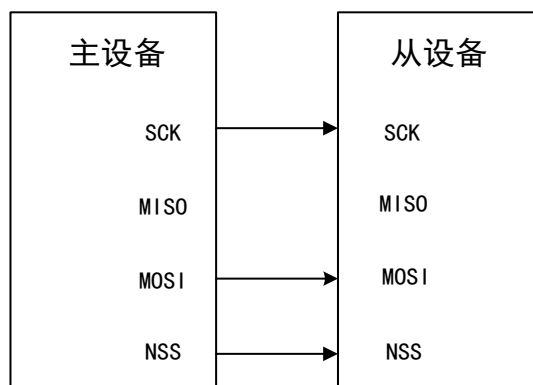
图 102 单工模式连接（主机只发送，从机接收）
