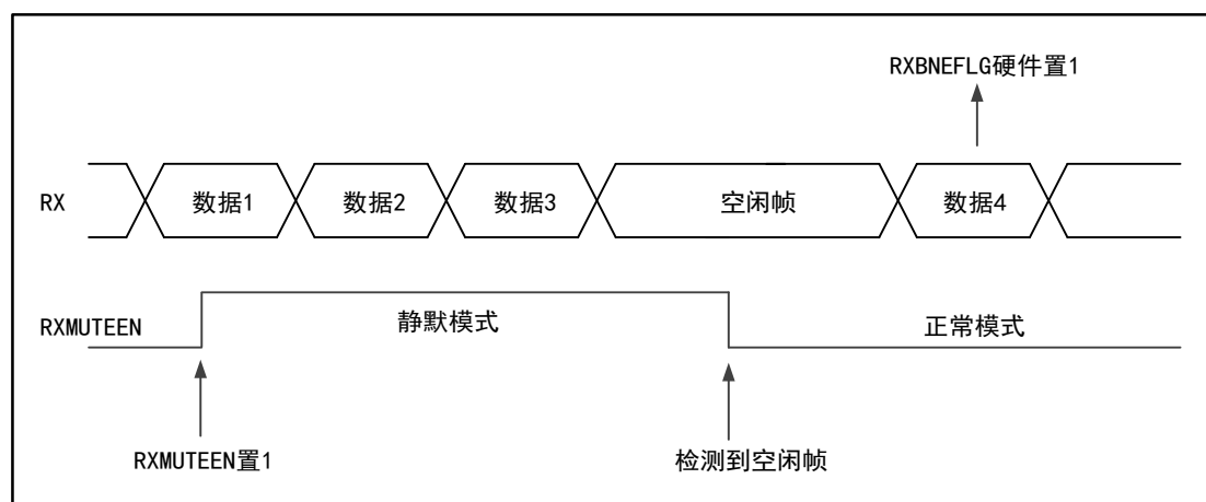
图 85 空闲总线退出静默模式
