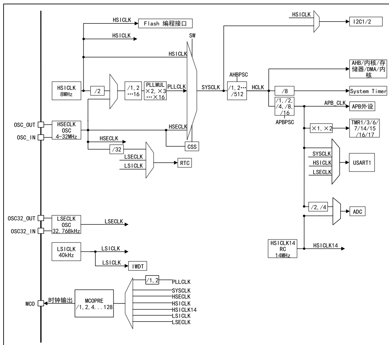
图 5 APM32F030xC 时钟树
