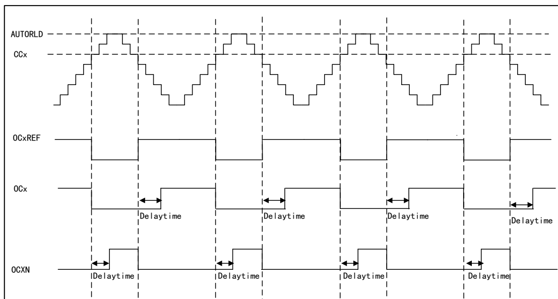
图 75 带死区插入的互补输出
