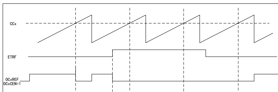
图 60 OCxREF 时序图
