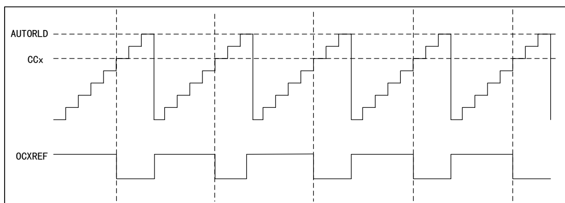
图 63 PWM1 向上计数模式的时序图
