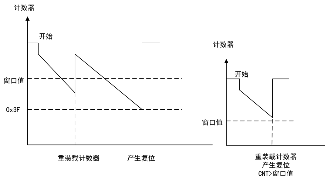
图 82 窗口看门狗时序图
