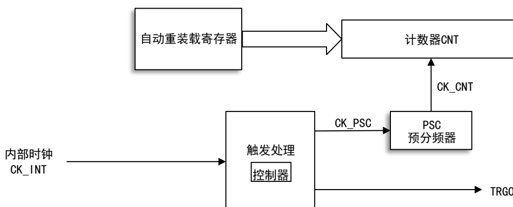
图 77 基本定时器结构框图
