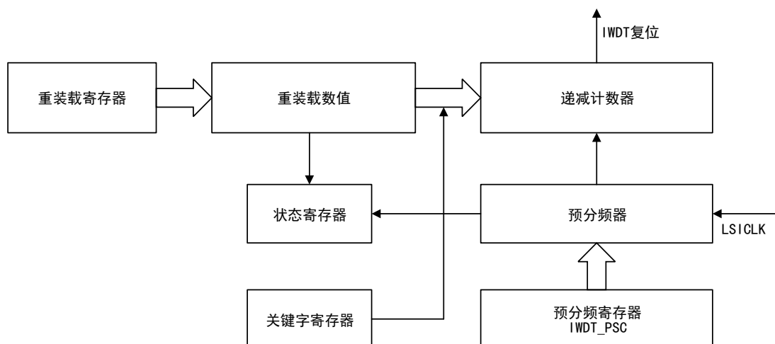
图 80 独立看门狗结构框图
