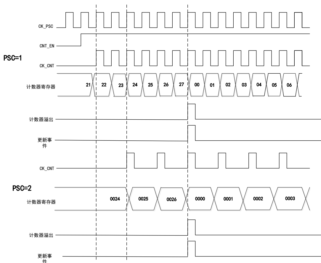
图 78 计数器时序图，内部时钟分频系数为 1 或 2
