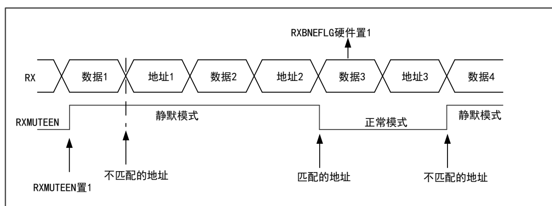
图 86 地址标记退出静默模式
