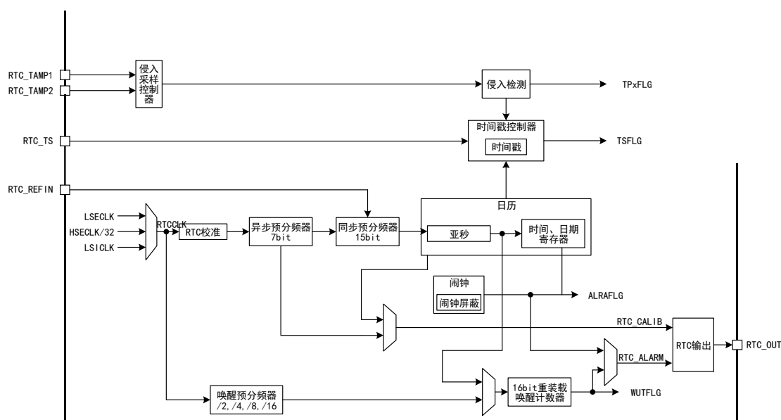
图 84 APM32F030xC RTC 结构框图
