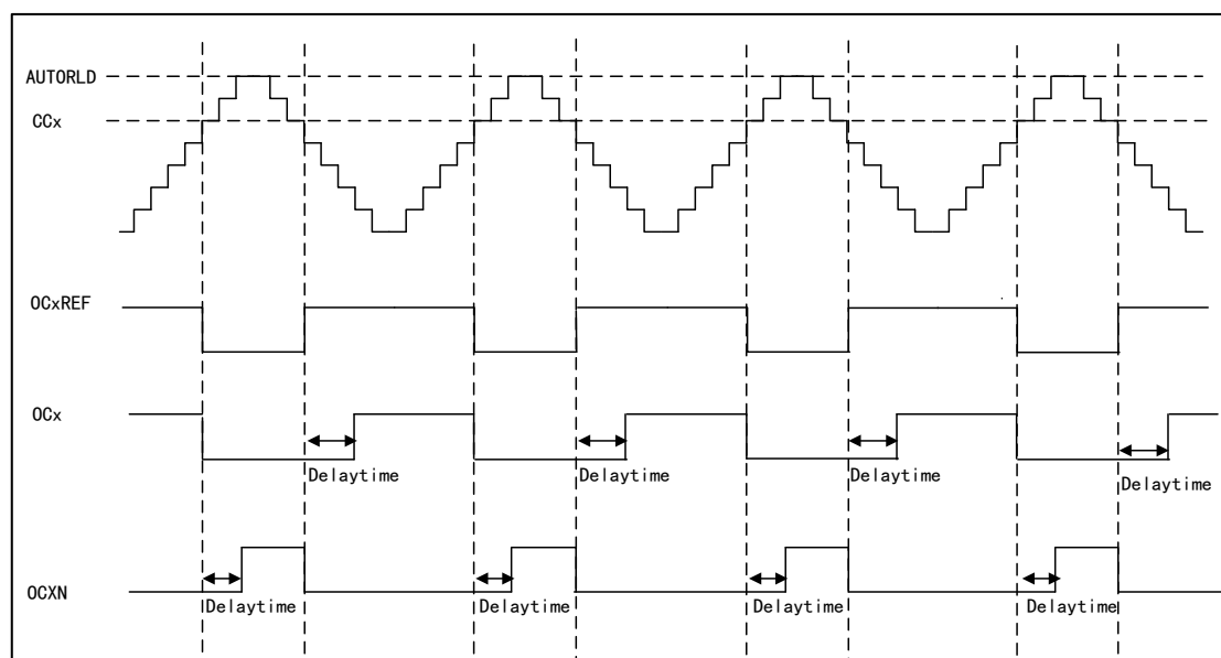
图 38 带死区插入的互补输出
