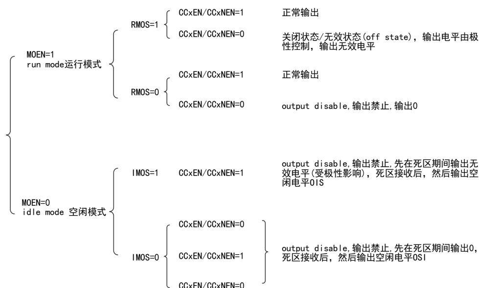
图 73 影响输出波形的寄存器结构关系
