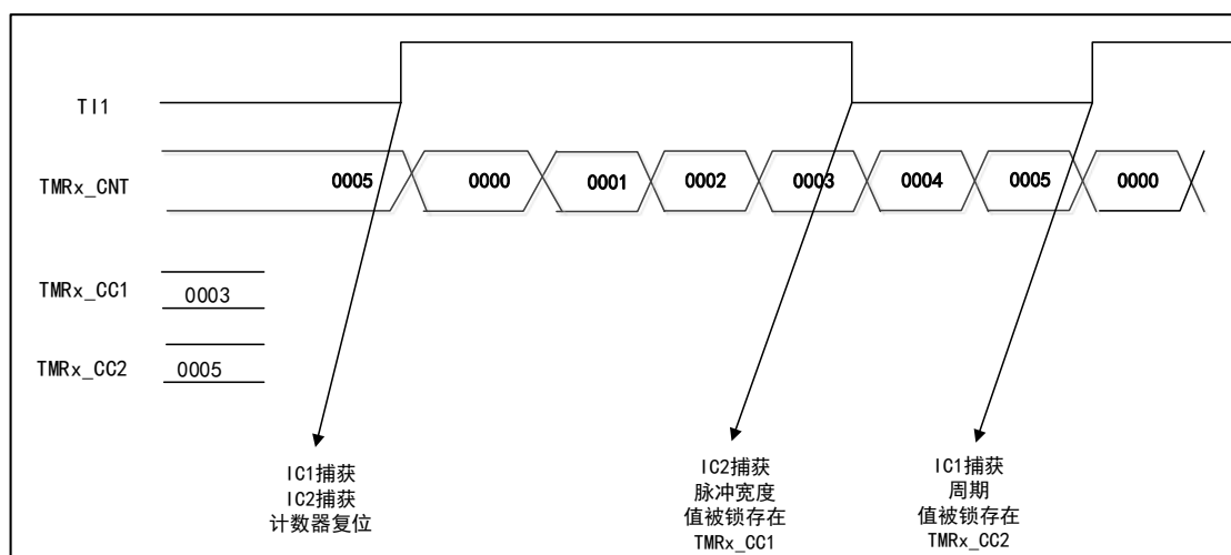
图 71 PWM 输入模式时序图
