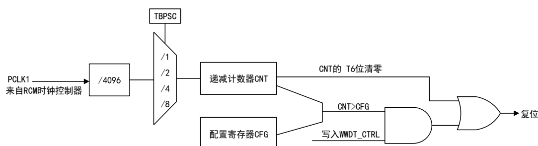
图 81 窗口看门狗结构框图
