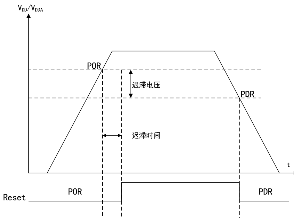
图 8 上电复位和掉电复位的波形图
