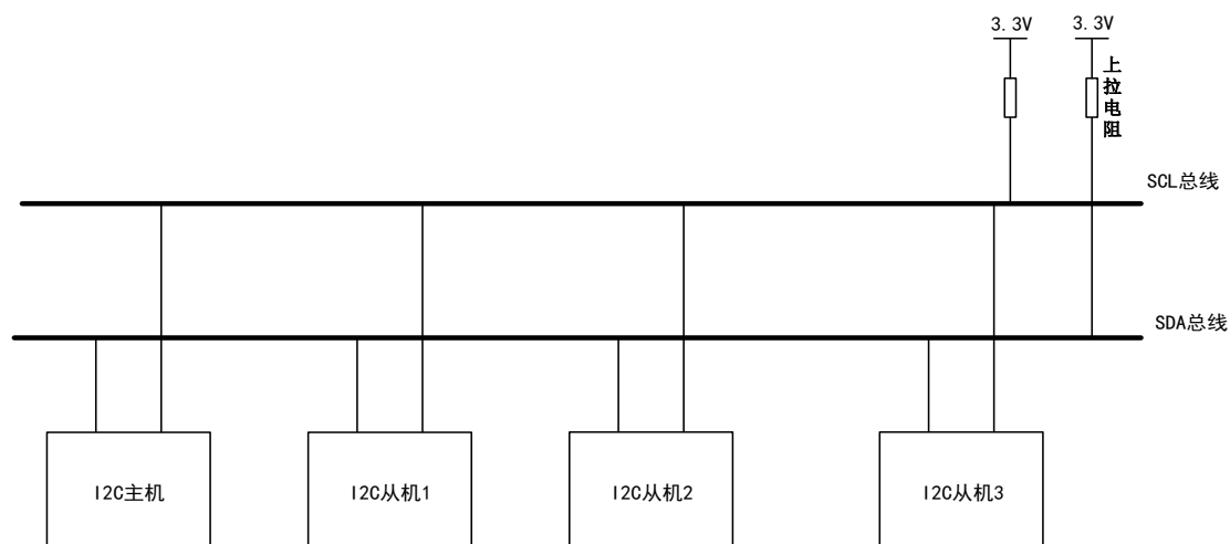
图 95 常见 I2C 通信连接图
