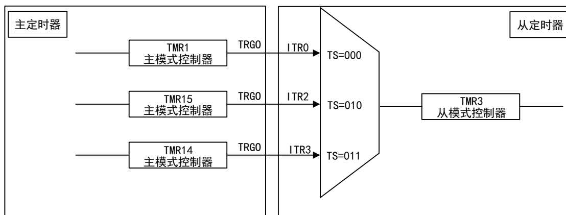
图 58 TMR3 与其它定时器互连
