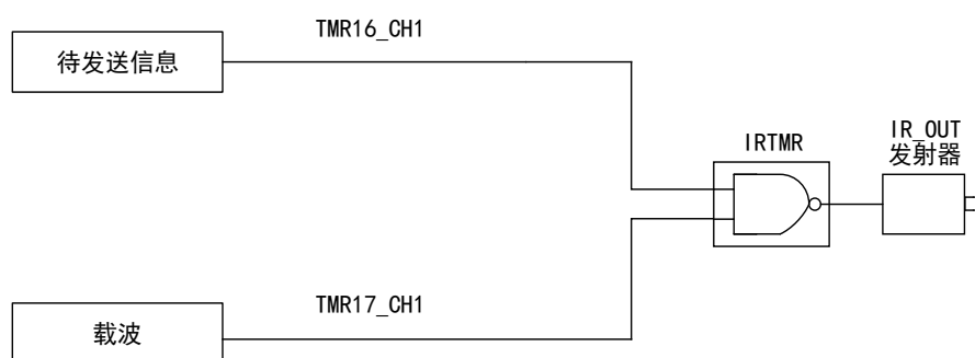
图 79 IRTMR 结构框图
