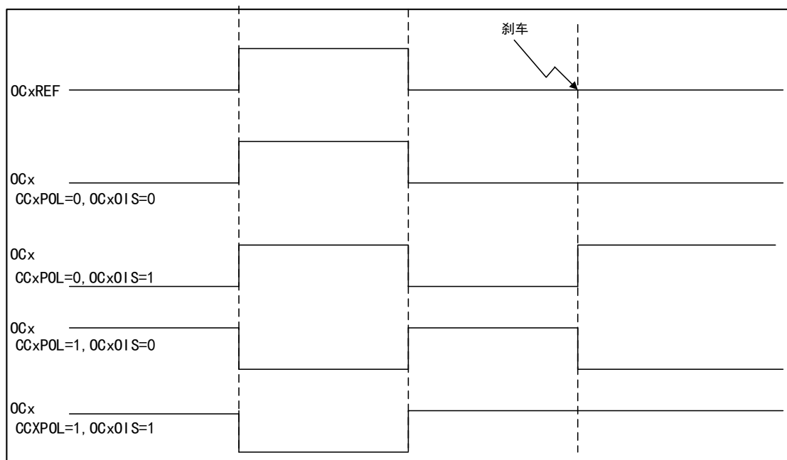
图 74 发生刹车事件的时序图
